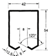
Tipo B 25/10 kg/m 3,18
