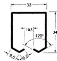
Tipo C 20/10 kg/m 1,77
