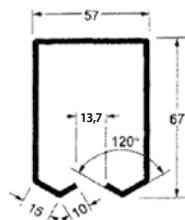
Tipo A 30/10 kg/m 5,00
